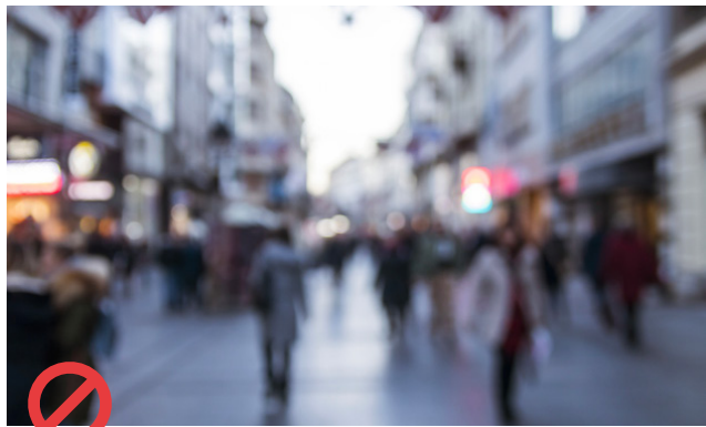
Blurry images
